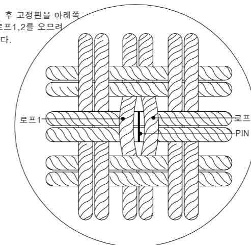
PIN 시공방법상세도
