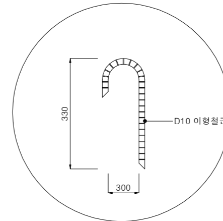
L형 고정핀 상세도
