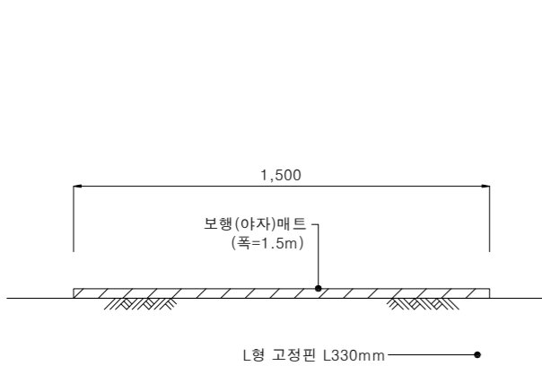
보행(야자)매트 단면도
